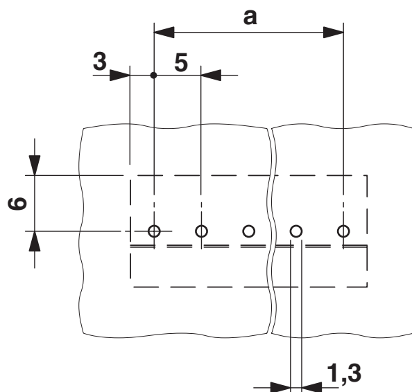
Borrplan/lödöns geometri
