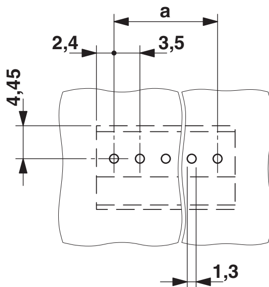
Borrplan/lödöns geometri
