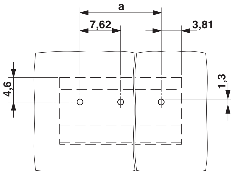
Borrplan/lödöns geometri
