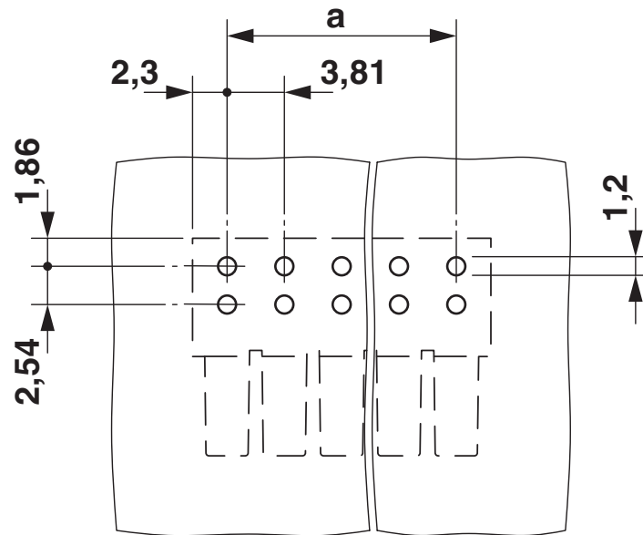
Borrplan/lödöns geometri
