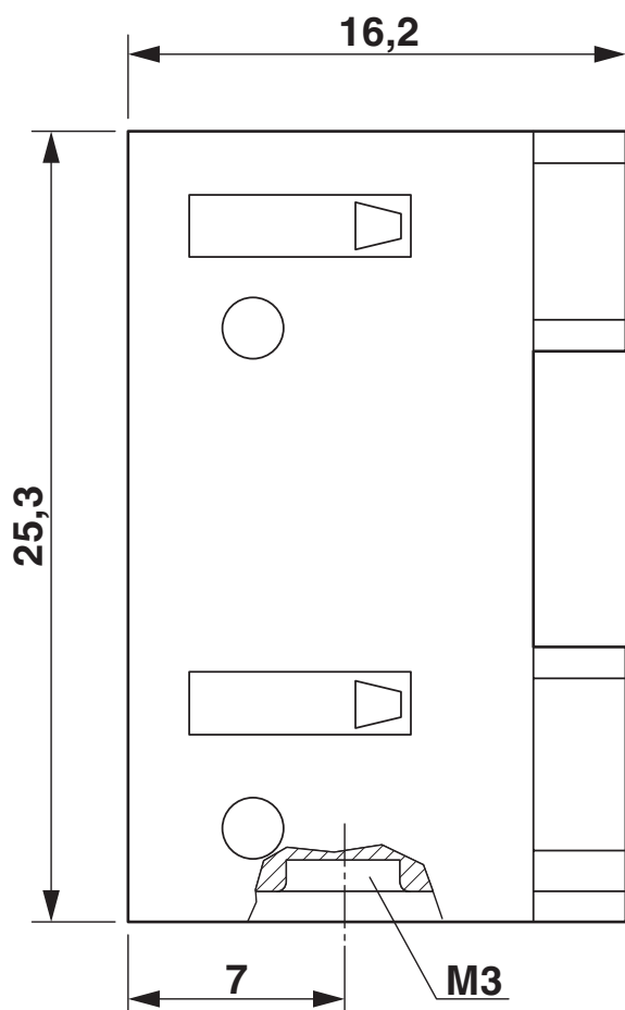
Måttskiss
