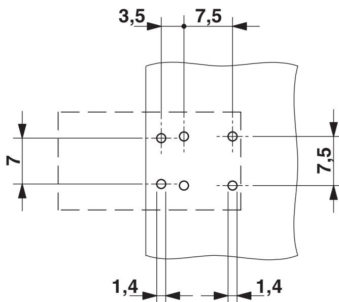
Borrplan/lödöns geometri
