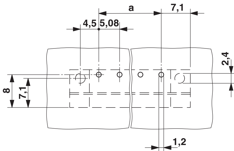
Borrplan/lödöns geometri
