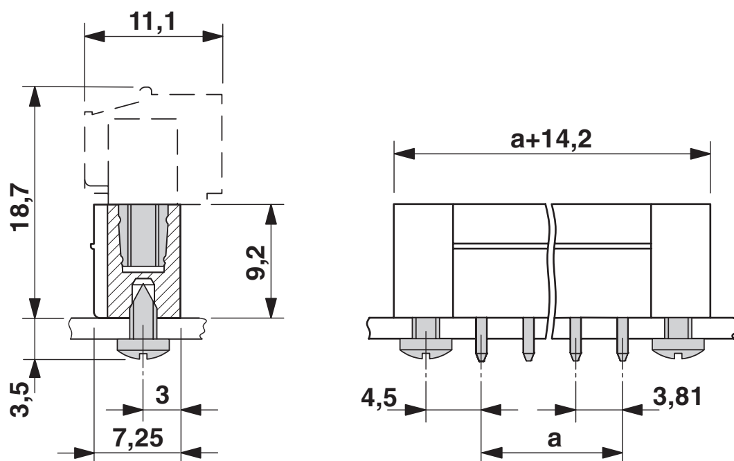
Måttskiss
