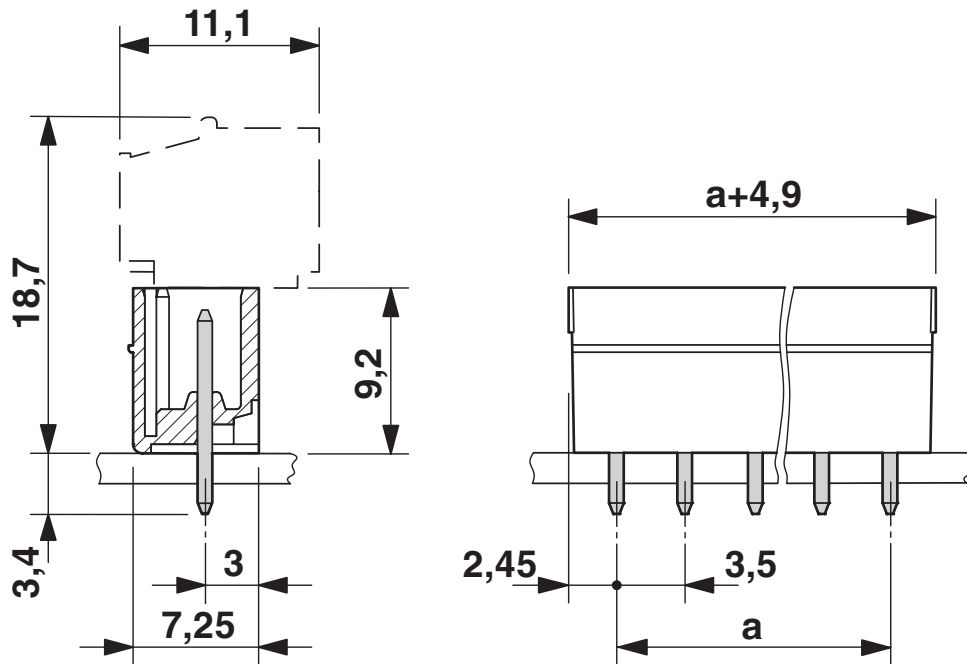
Måttskiss
