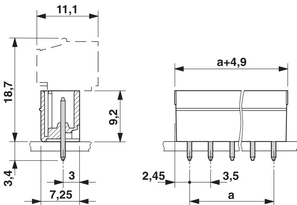
Måttskiss
