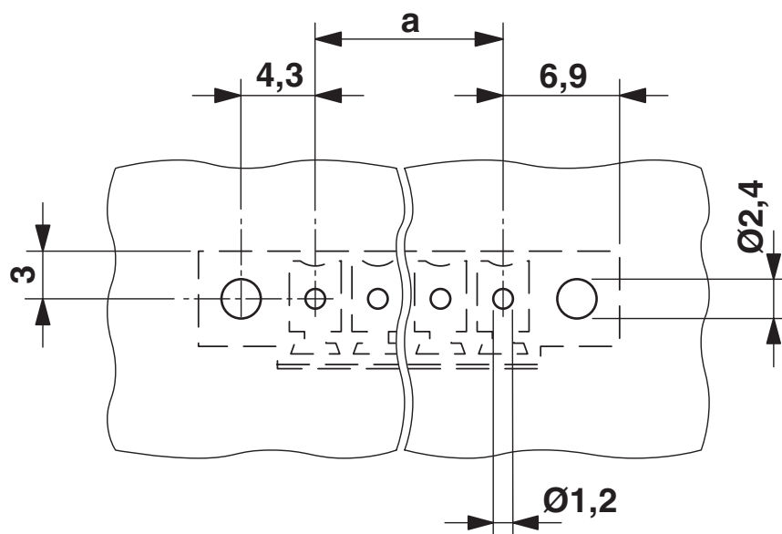
Borrplan/lödöns geometri
