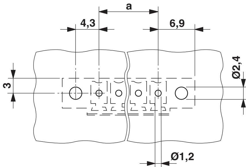
Borrplan/lödöns geometri
