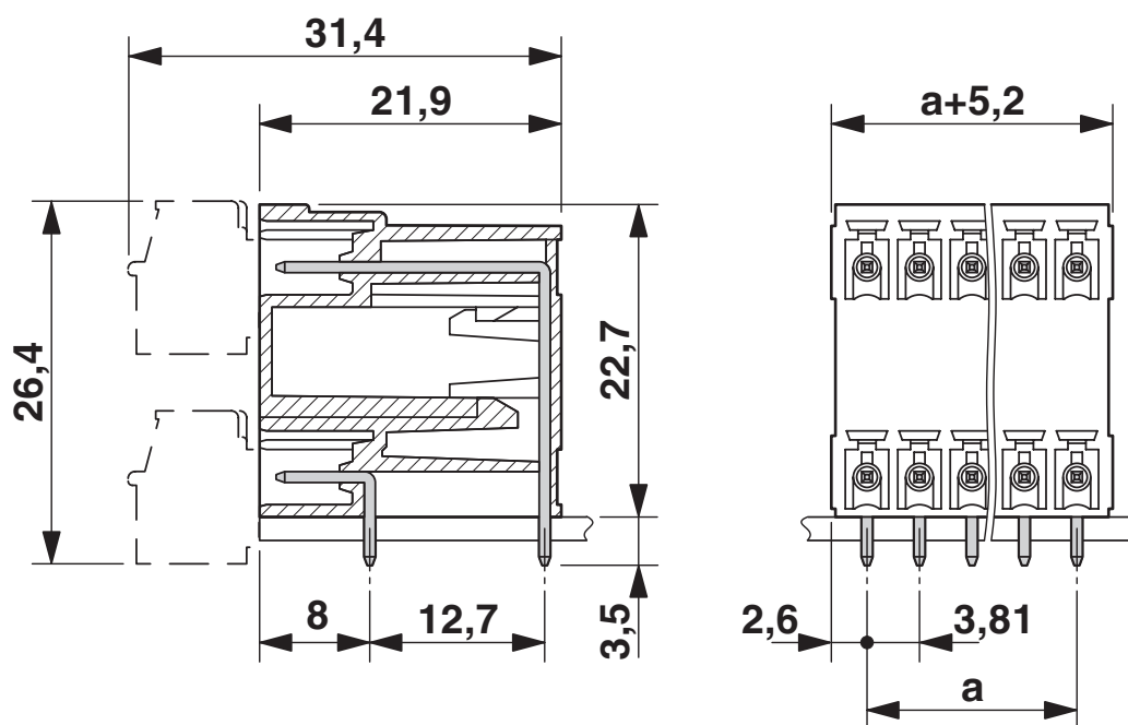
Måttskiss
