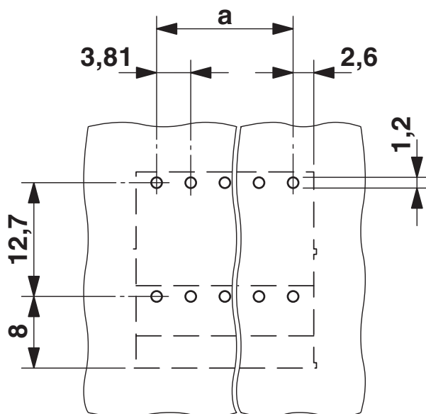
Borrplan/lödöns geometri
