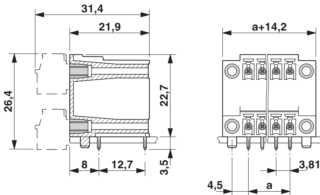
Måttskiss
