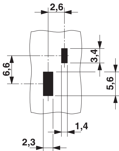
Borrplan/lödöns geometri
