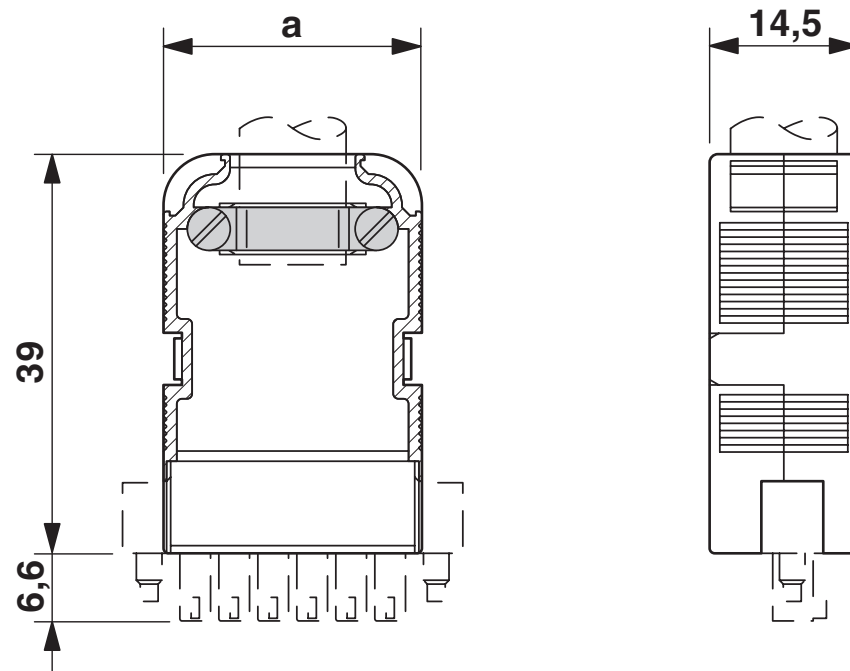
Måttskiss
