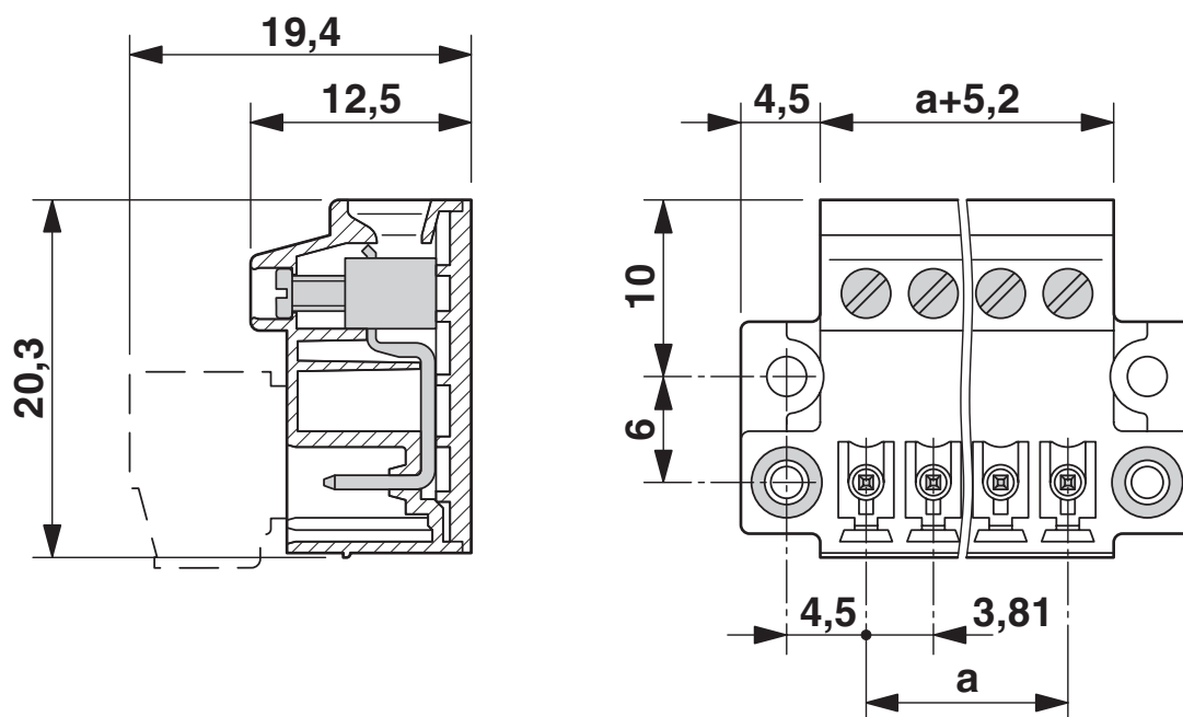
Måttskiss
