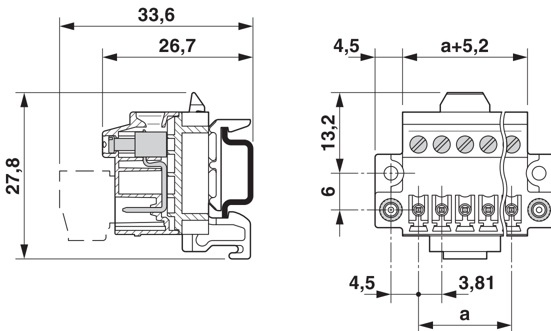
Måttskiss
