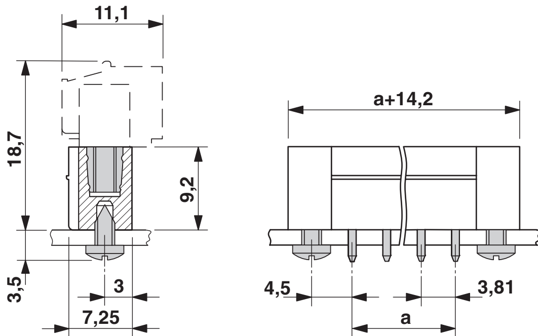
Måttskiss
