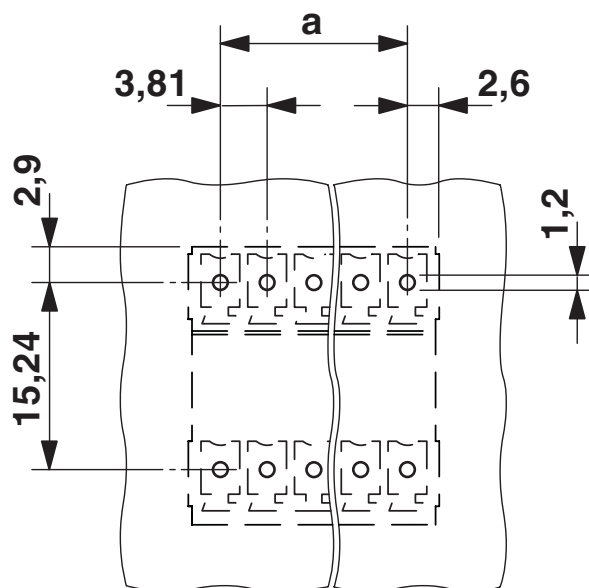
Borrplan/lödöns geometri
