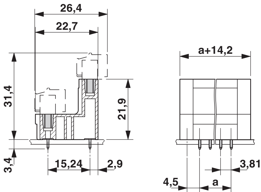
Måttskiss
