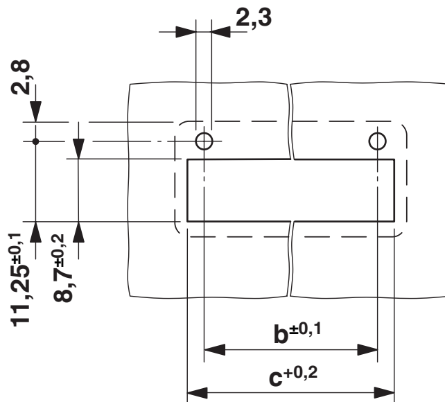
Borrplan/lödöns geometri
