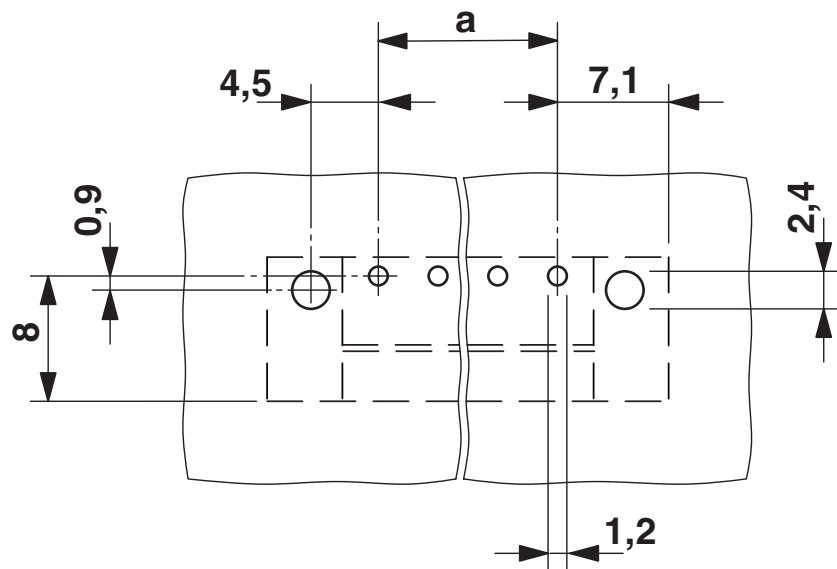
Borrplan/lödöns geometri
