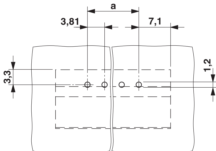
Borrplan/lödöns geometri
