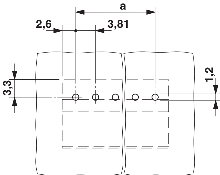
Borrplan/lödöns geometri
