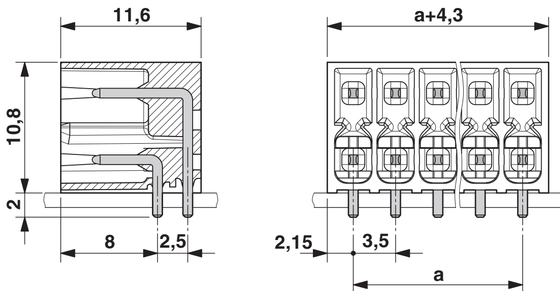
Schematisk ritning
