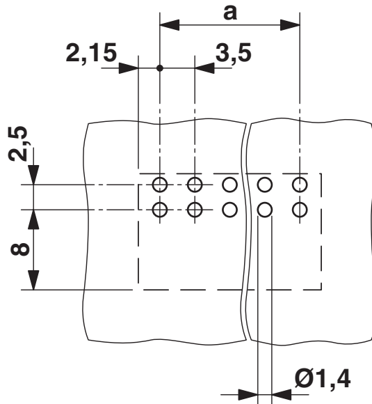
Borrplan/lödöns geometri
