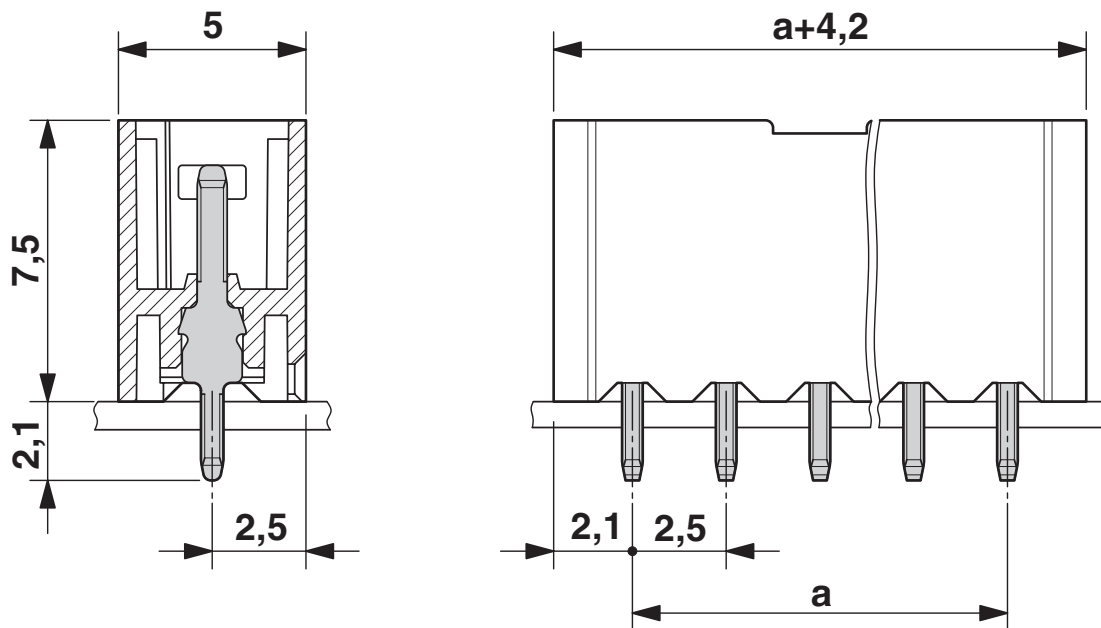
Måttskiss
