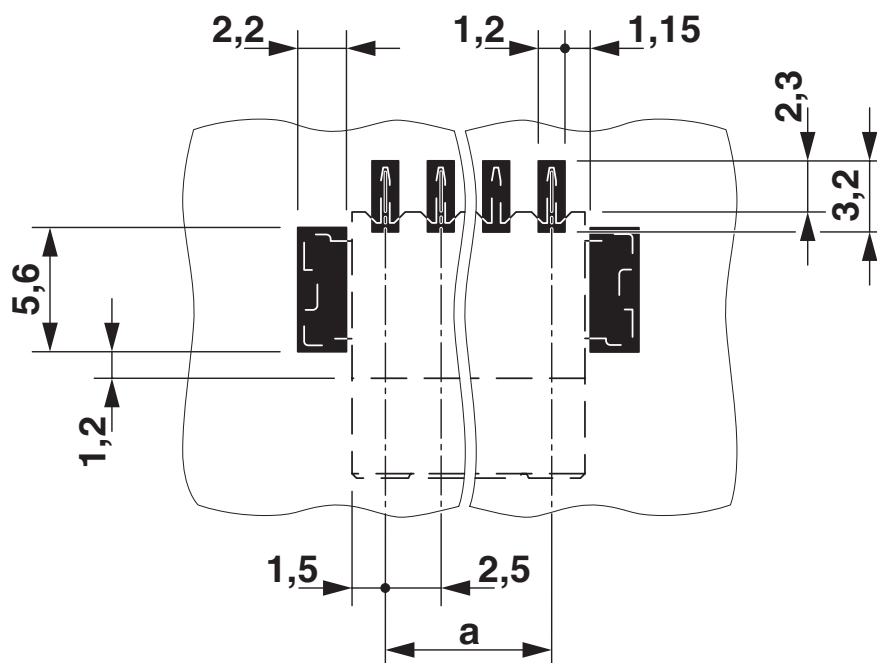
Borrplan/lödöns geometri
