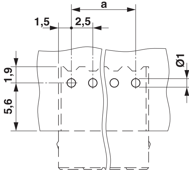
Borrplan/lödöns geometri
