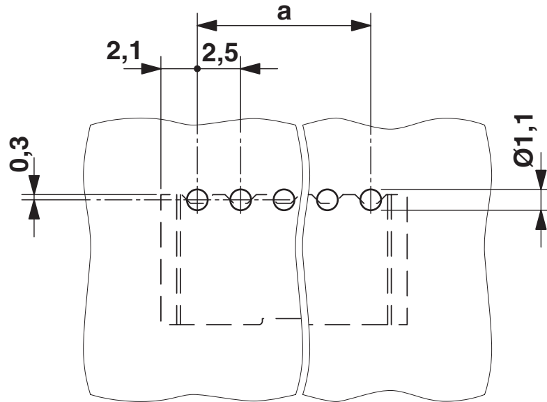
Borrplan/lödöns geometri
