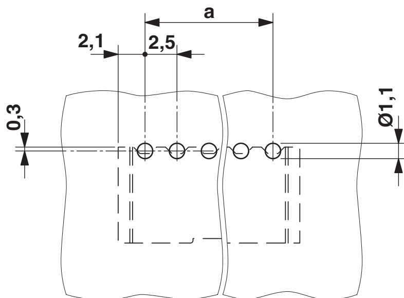
Borrplan/lödöns geometri
