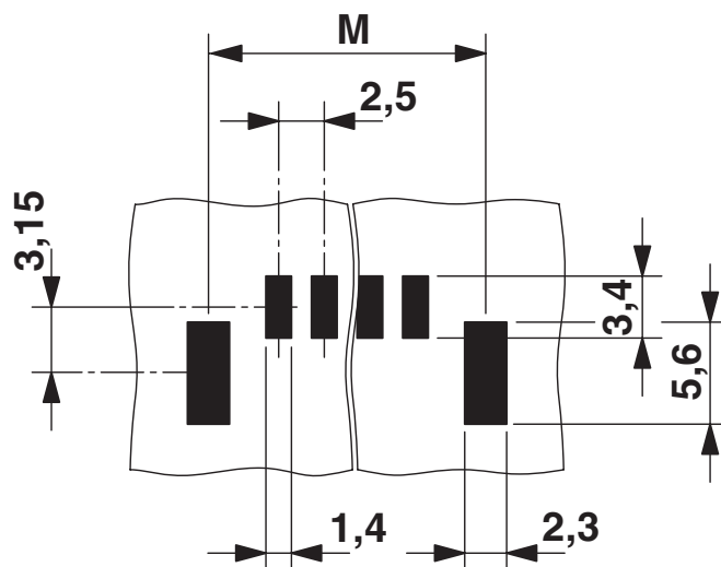
Borrplan/lödöns geometri
