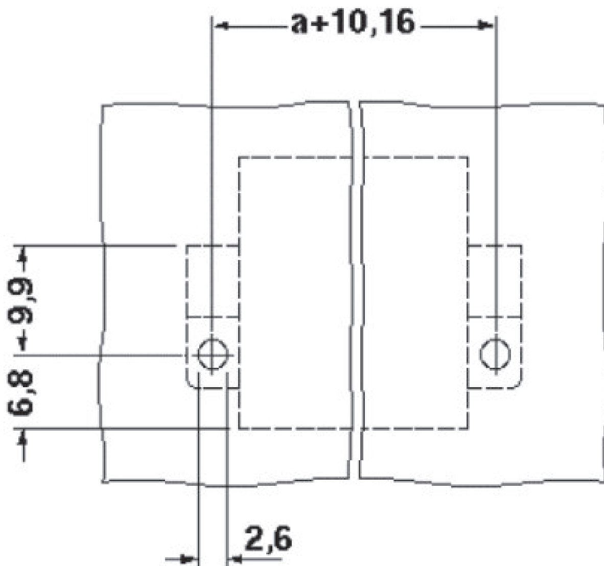
Borrplan/lödöns geometri
