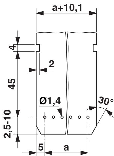
Borrplan/lödöns geometri
