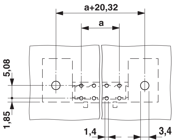
Borrplan/lödöns geometri
