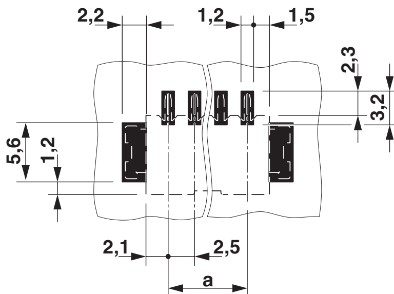
Borrplan/lödöns geometri
