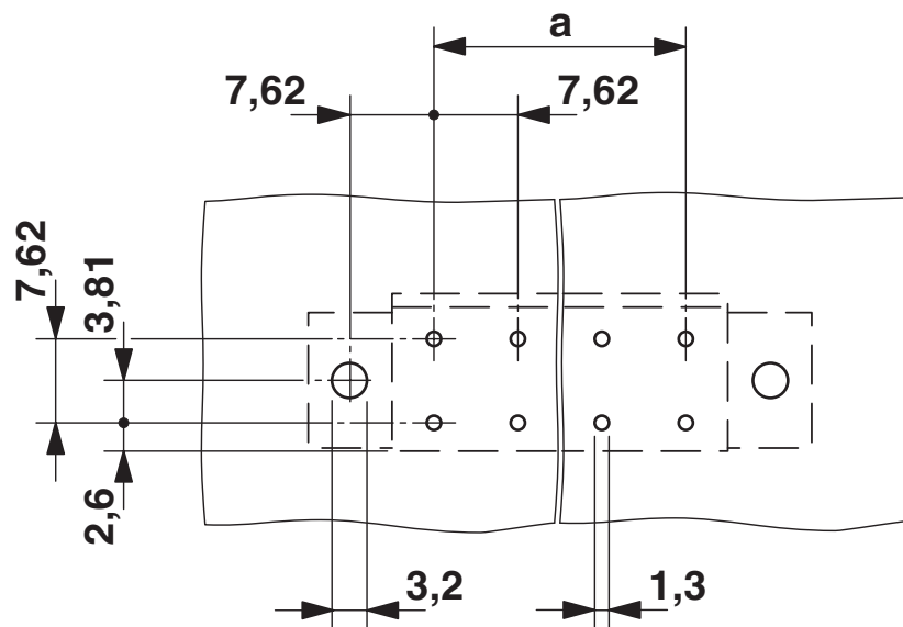
Borrplan/lödöns geometri
