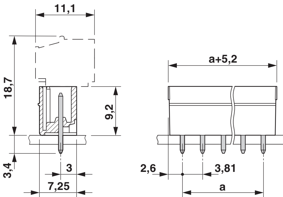
Måttskiss
