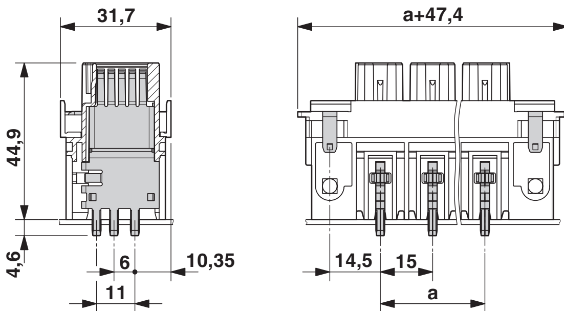
Måttskiss
