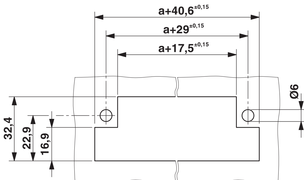
Måttskiss
