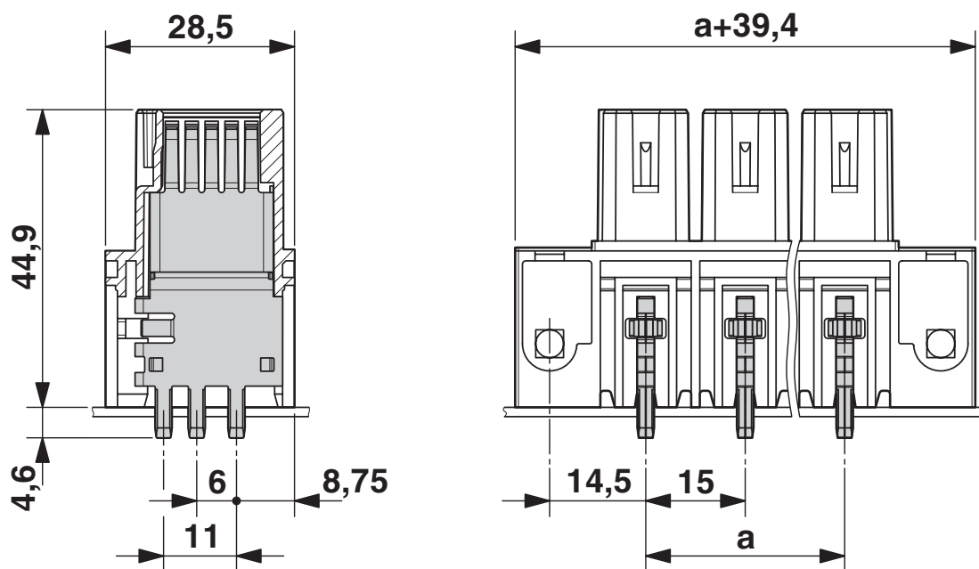
Måttskiss
