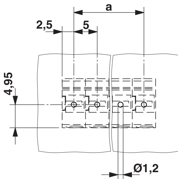
Borrplan/lödöns geometri
