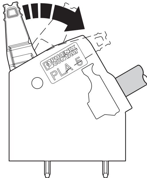
Funktionsritning
