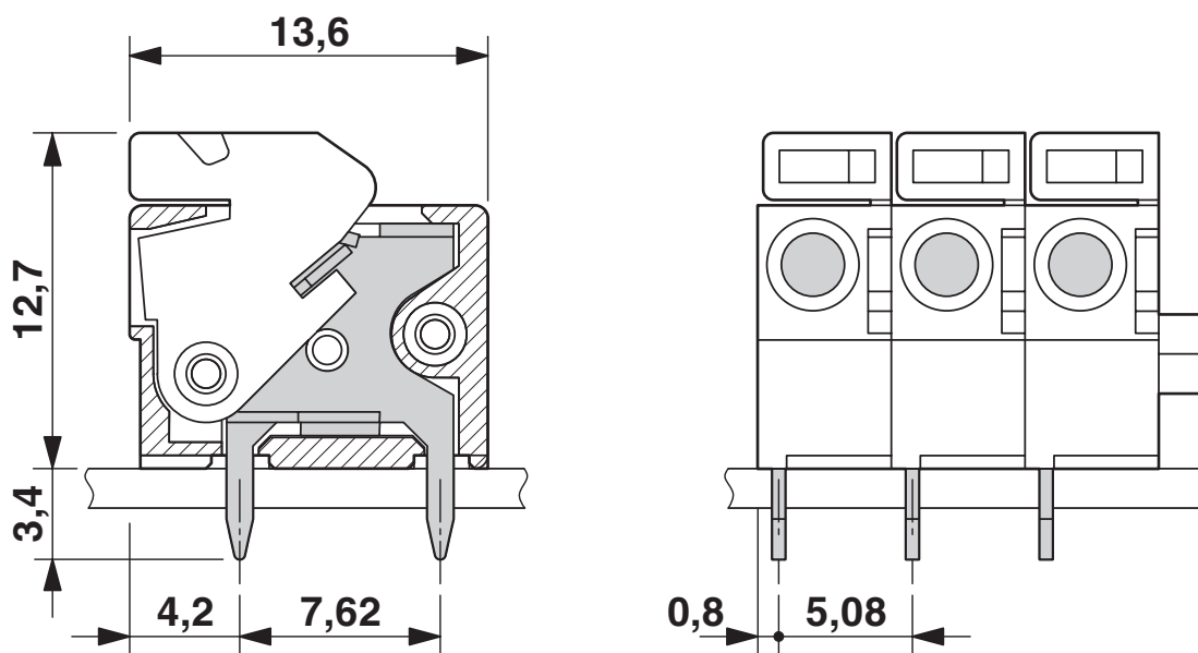
Måttskiss
