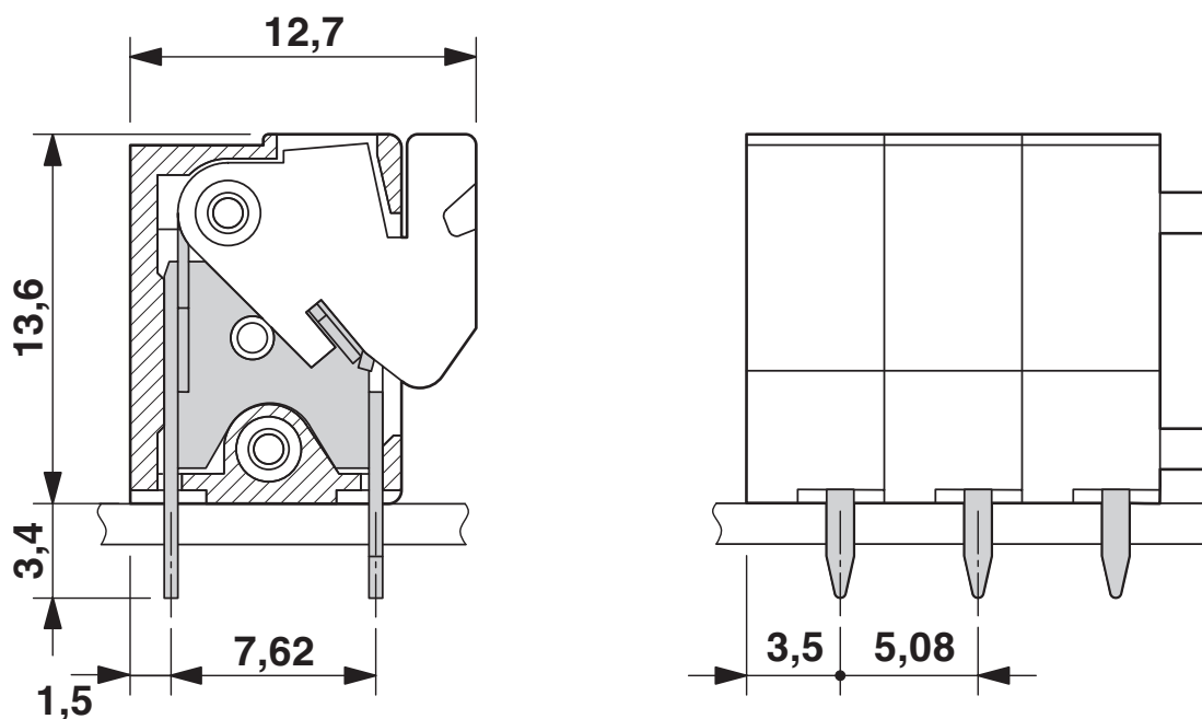
Måttskiss
