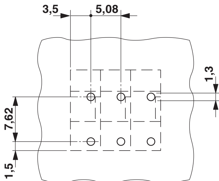
Borrplan/lödöns geometri
