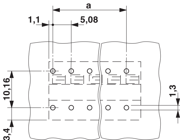
Borrplan/lödöns geometri
