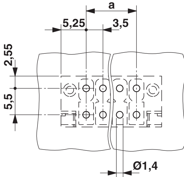
Borrplan/lödöns geometri
