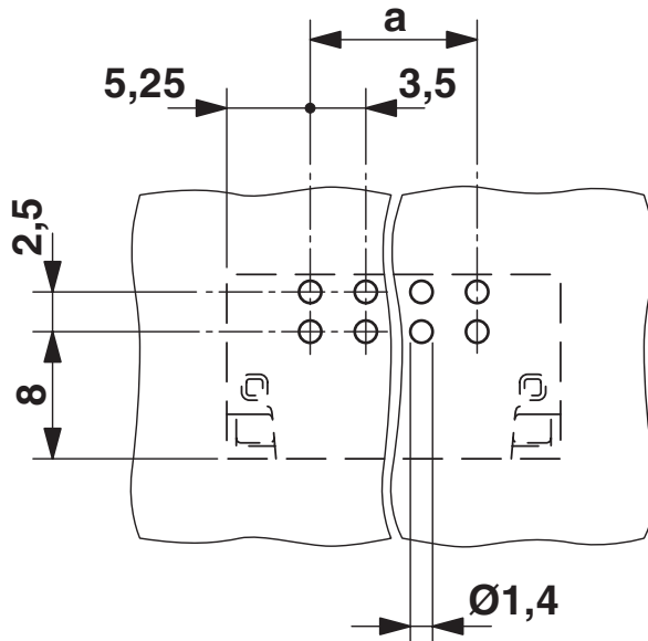
Borrplan/lödöns geometri
