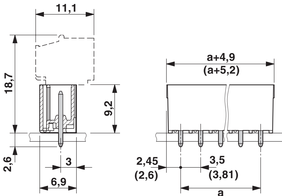
Måttskiss
