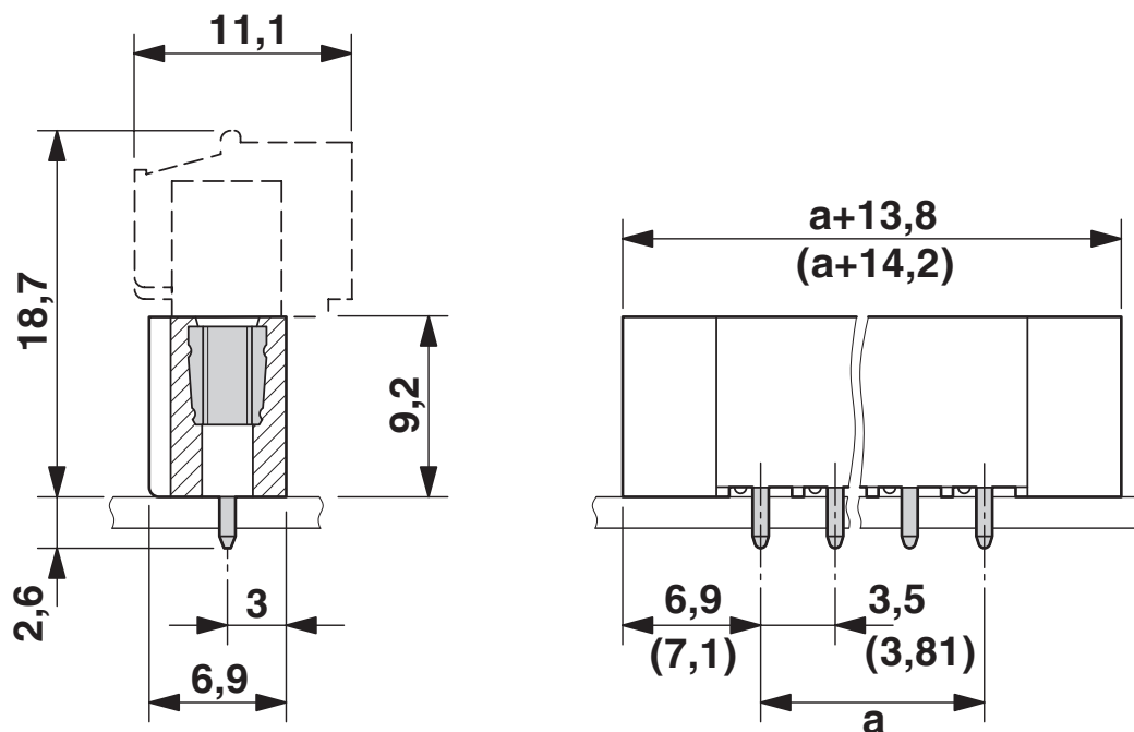
Måttskiss
