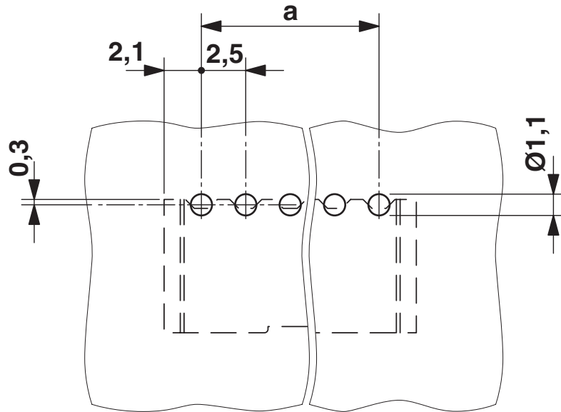
Borrplan/lödöns geometri
