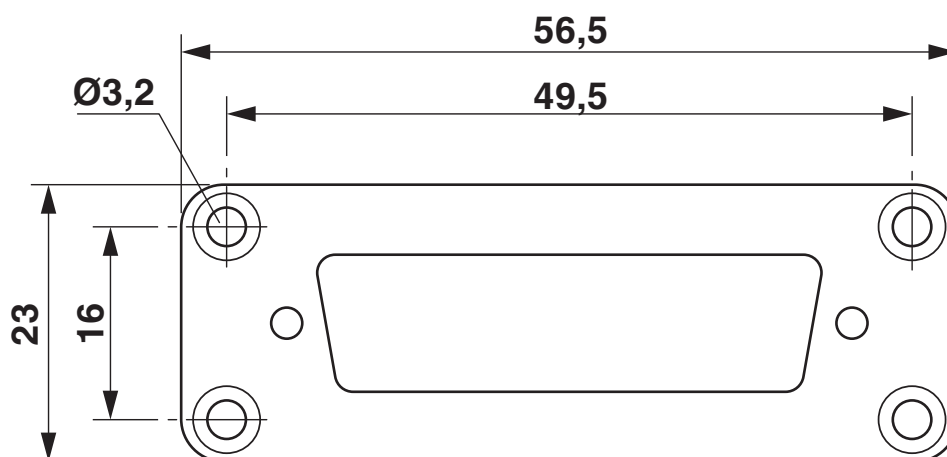
Måttskiss
